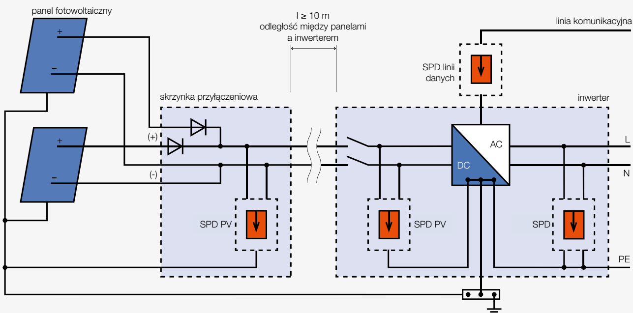
Podstawowy schemat okablowania i połączeń systemu fotowoltaicznego
